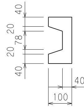
A-A断面
