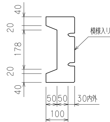
A-A断面
