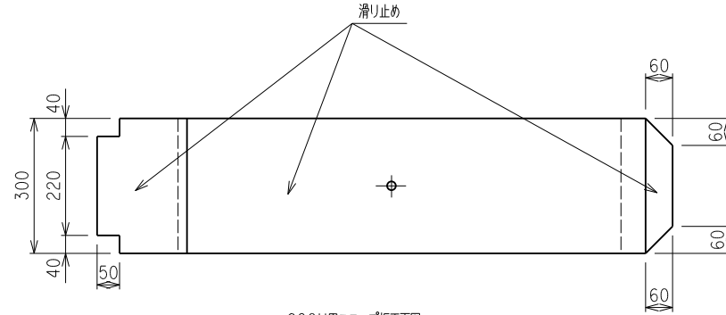
600H用スロープ板正面図
