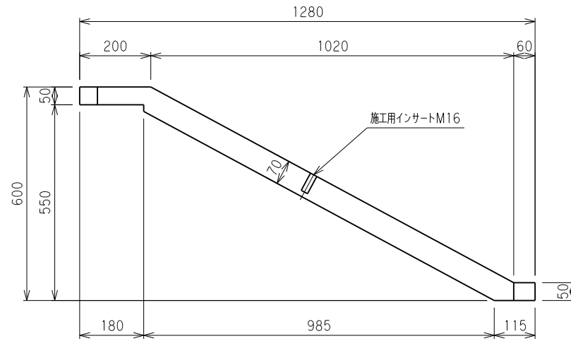
600H用スロープ板正面図
