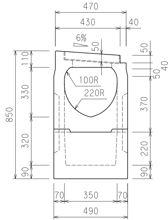
断面図
