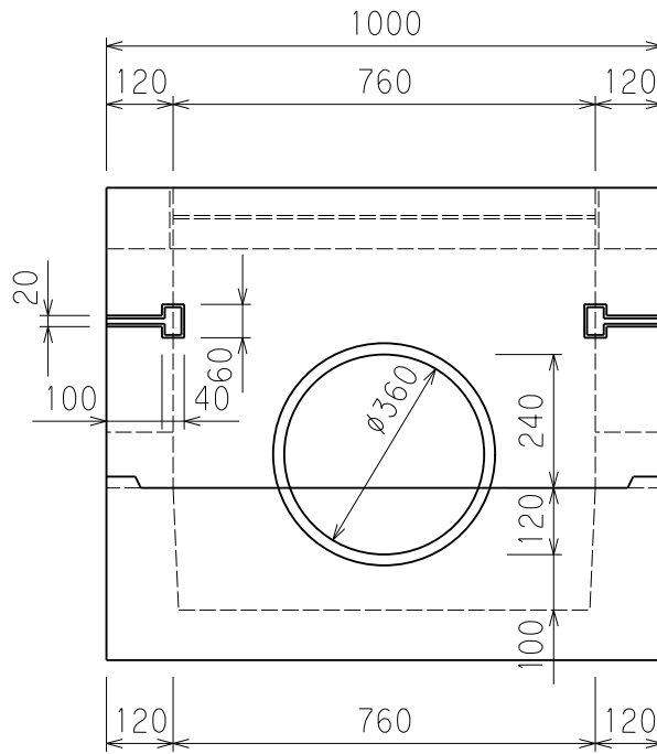
側面図
