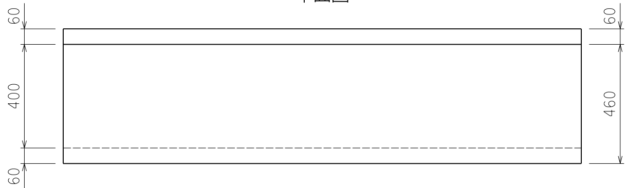
平面図
