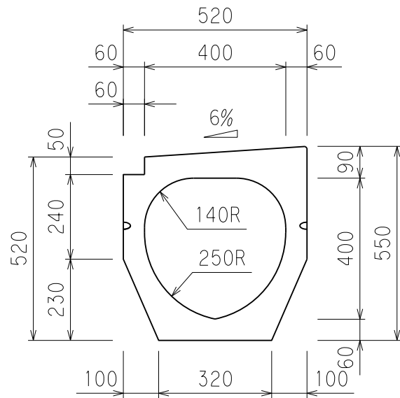
断面図
