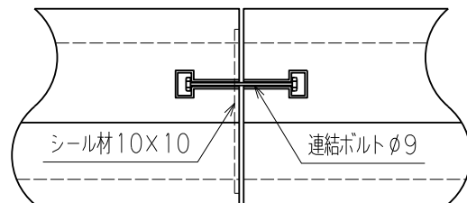
側面連結部
