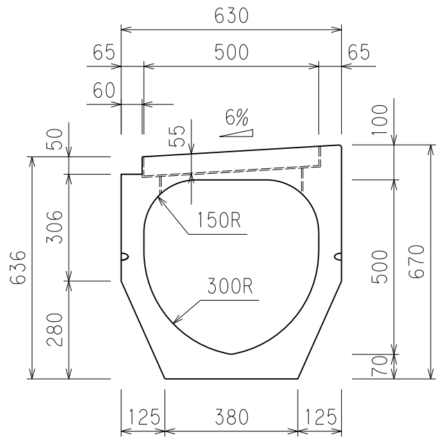
断面図
