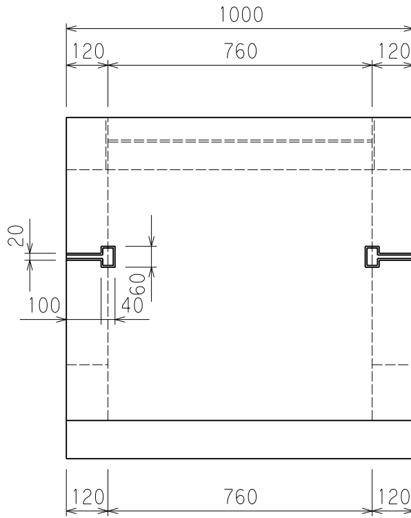
側面図
