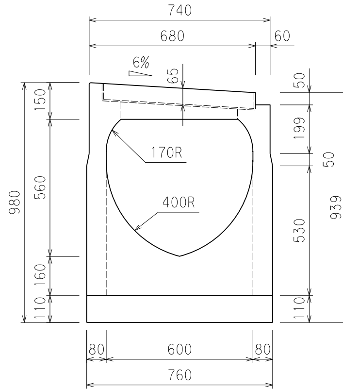
断面図
