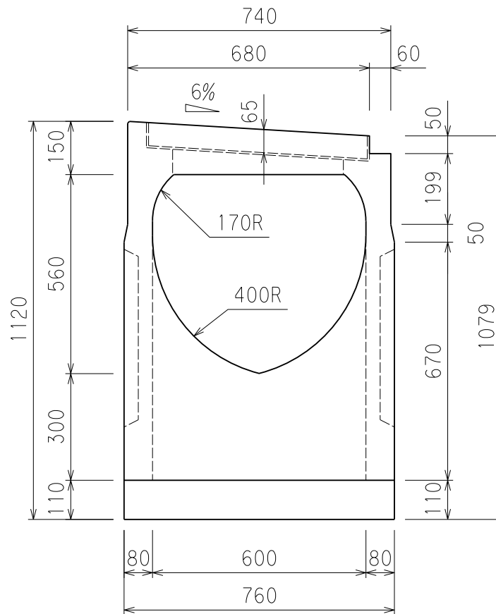
断面図
