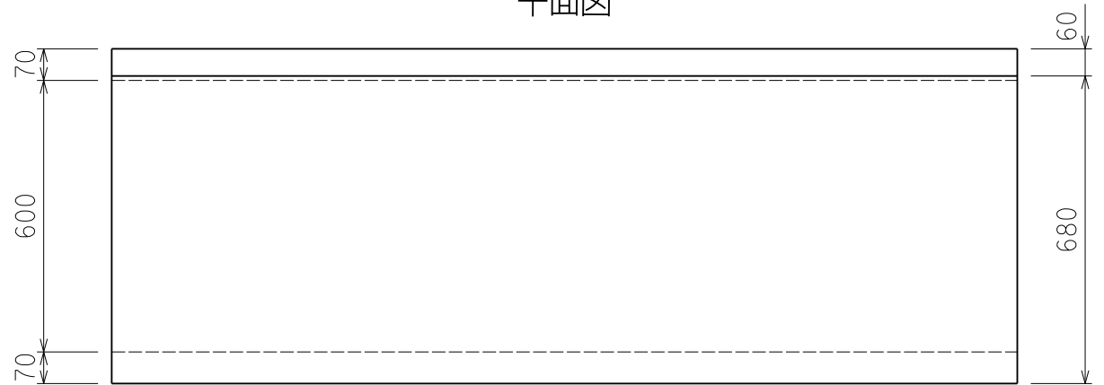
平面図
