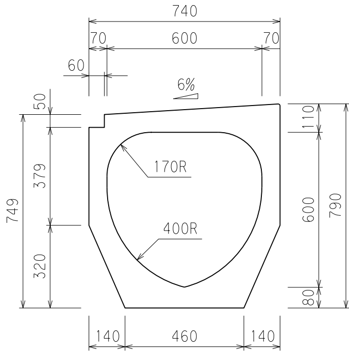
断面図
