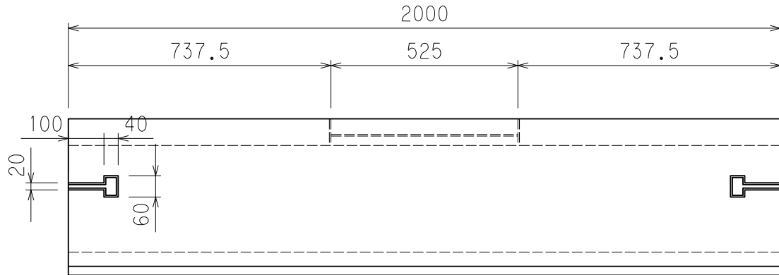
側面図
