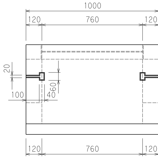
側面図
