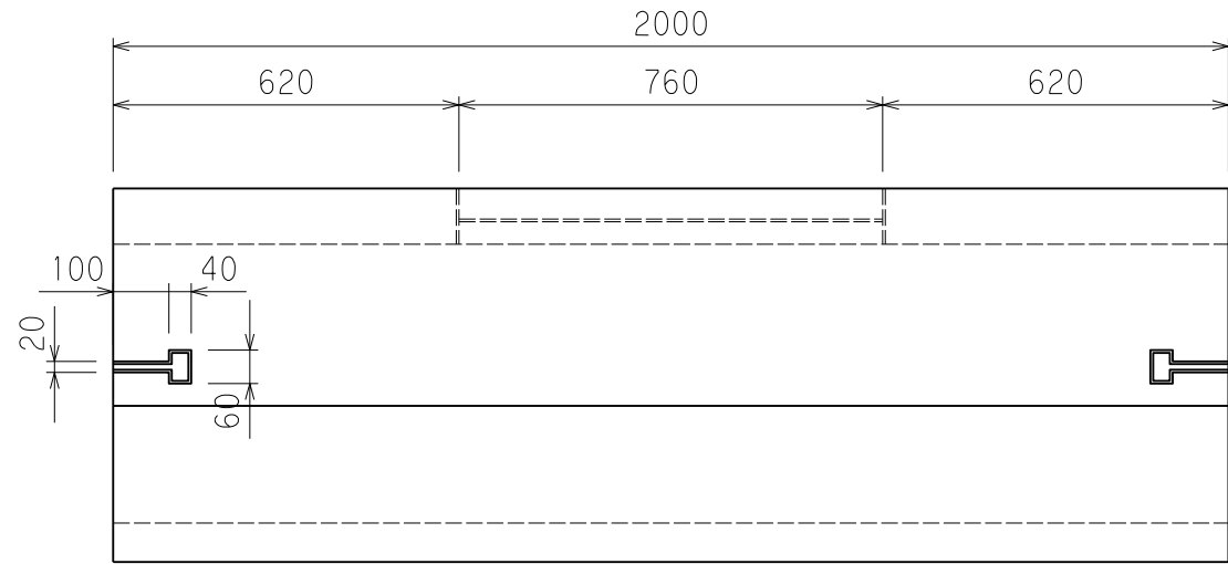
側面図
