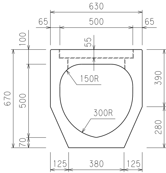
断面図
