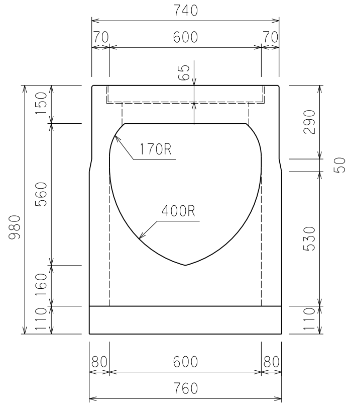
断面図
