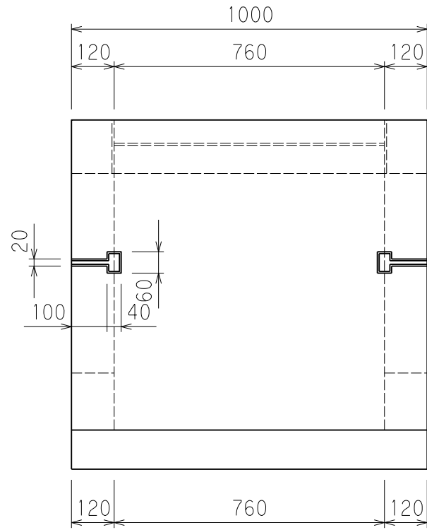
平面図
