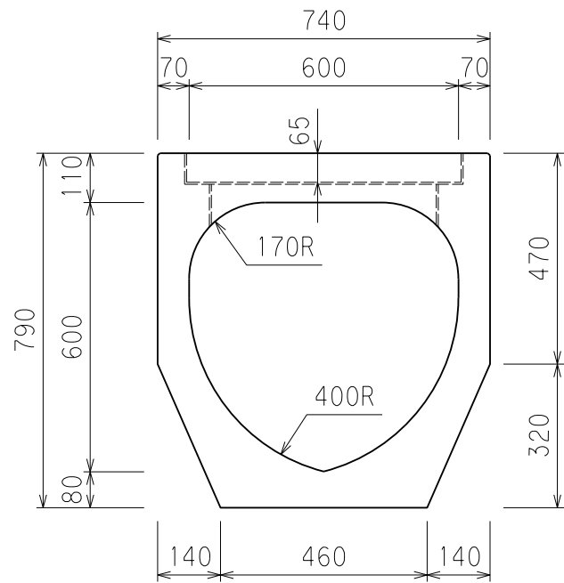
断面図
