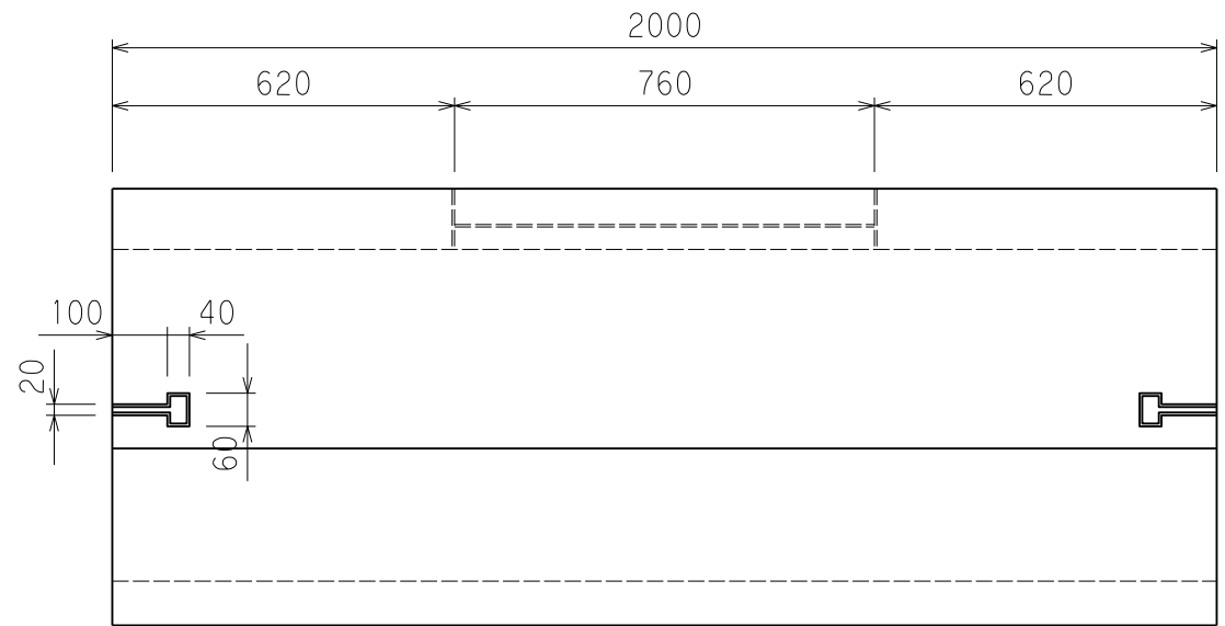
側面図
