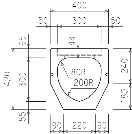
断面図
