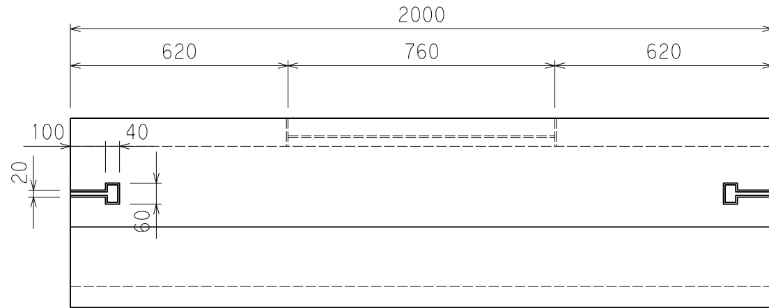
側面図
