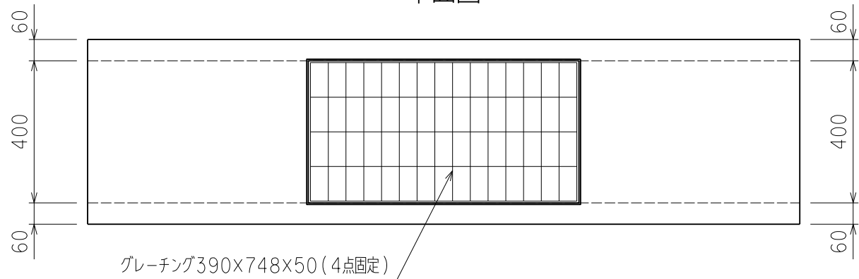
平面図
