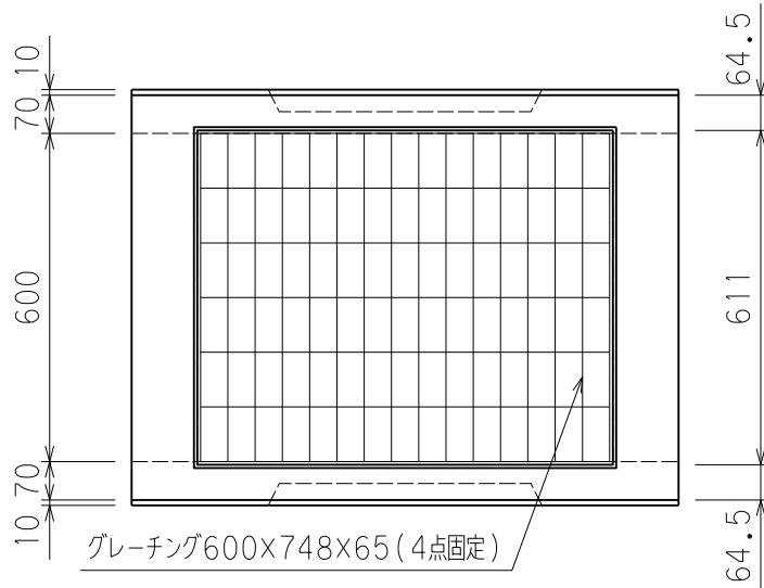
平面図
