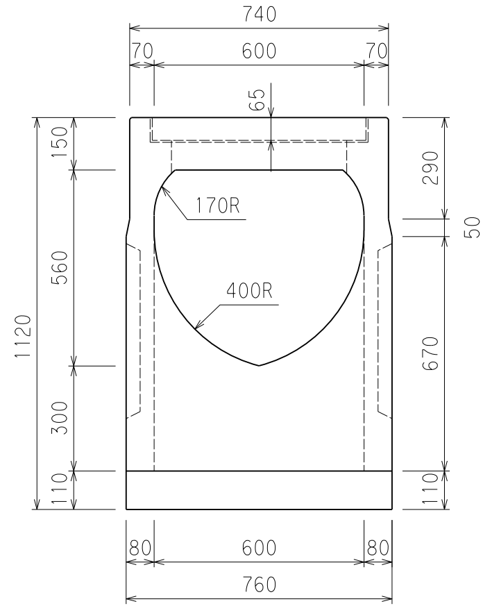
断面図
