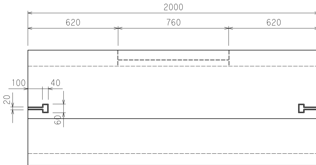
平面図
