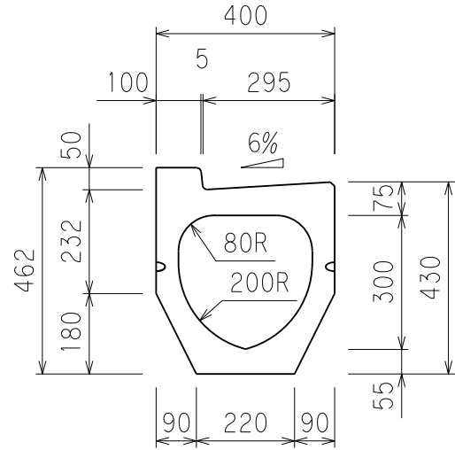
断面図
