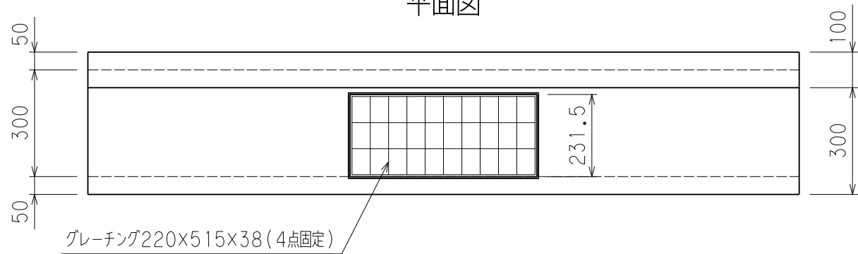
平面図
