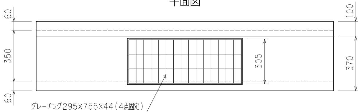
平面図
