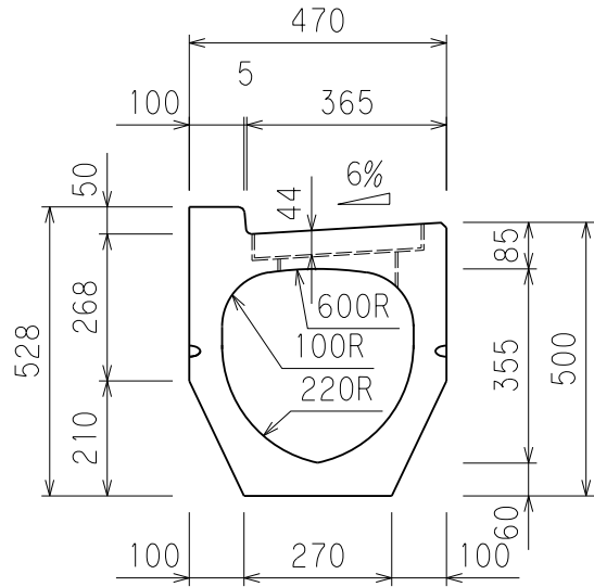
断面図
