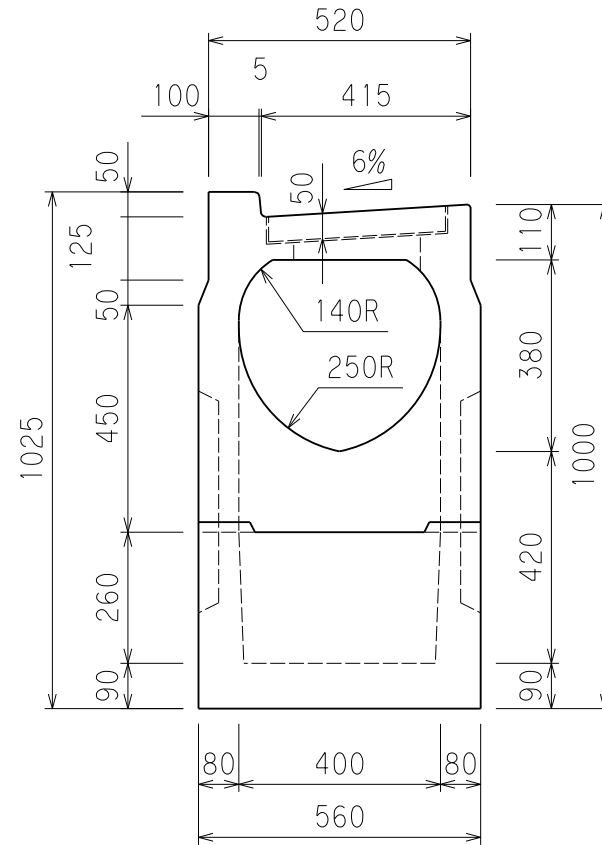
断面図
