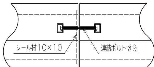
側面連結部
