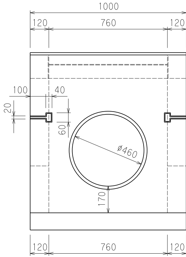
側面図
