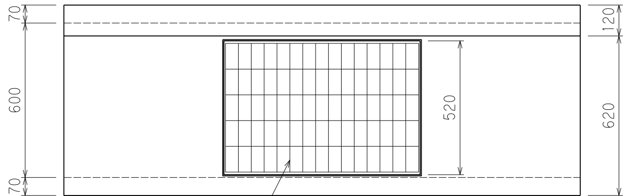
平面図
