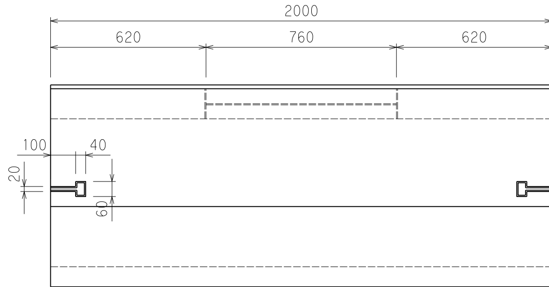
平面図
