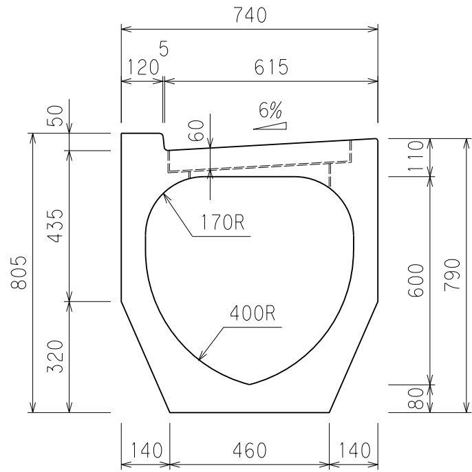
断面図
