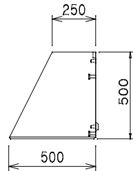
側面図(表)
