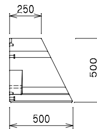
側面図(裏)
