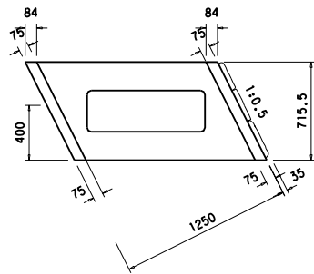
A-A 断面図
