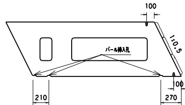
B-B 断面図
