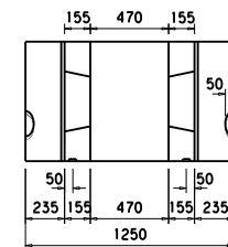
D-D 断面図
