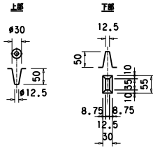
ガイドピン孔詳細 (S=1/10)
