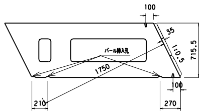
A-A 断面図
