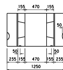
D-D 断面図
