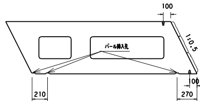
B-B 断面図
