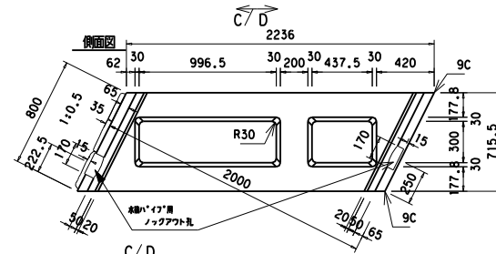
C/D 断面図
