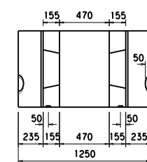
D-D 断面図
