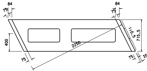
A-A 断面図
