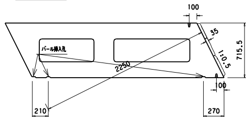
A-A 断面図
