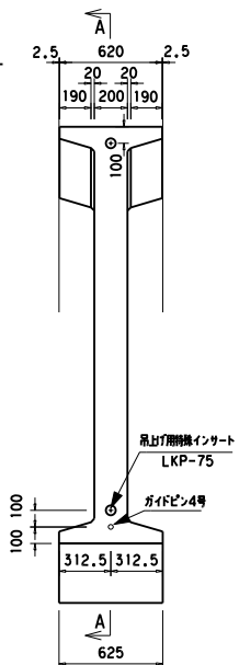
正面図
