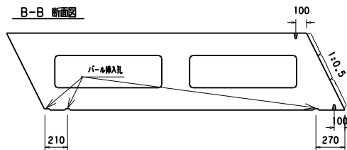
B-B 断面図
