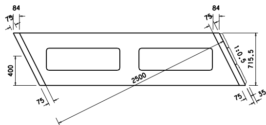
A-A 断面図
