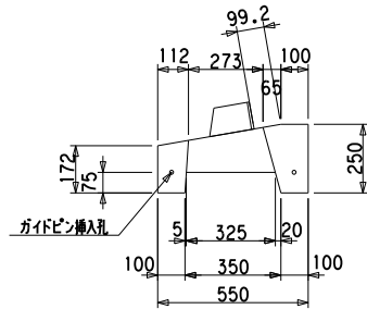
側面図
