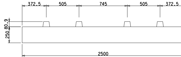
正面図
