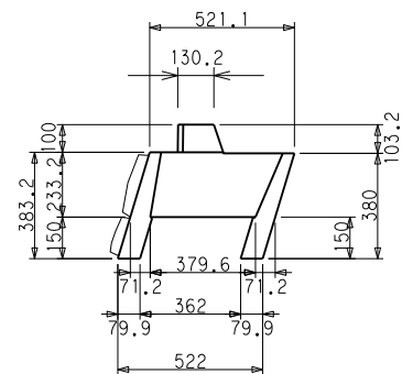
A-A断面図
