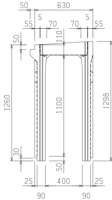
断面図
