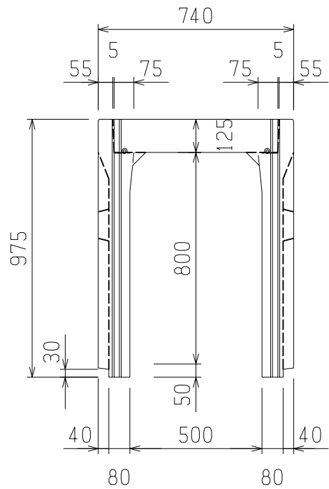
断面図
