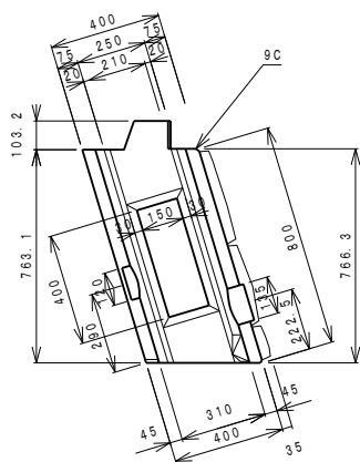
側面図
