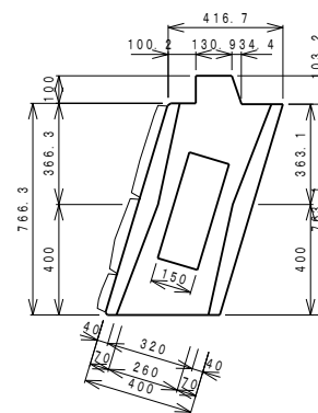
A-A断面図
