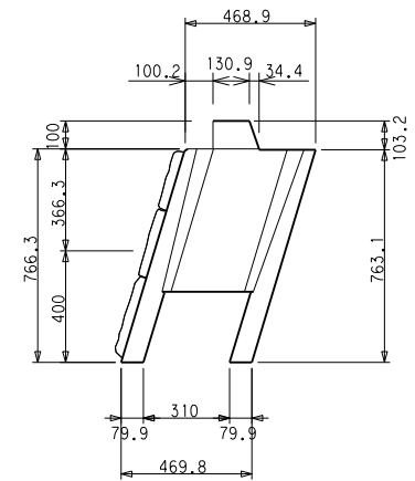
A-A断面図
