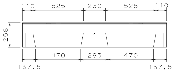
背面図
